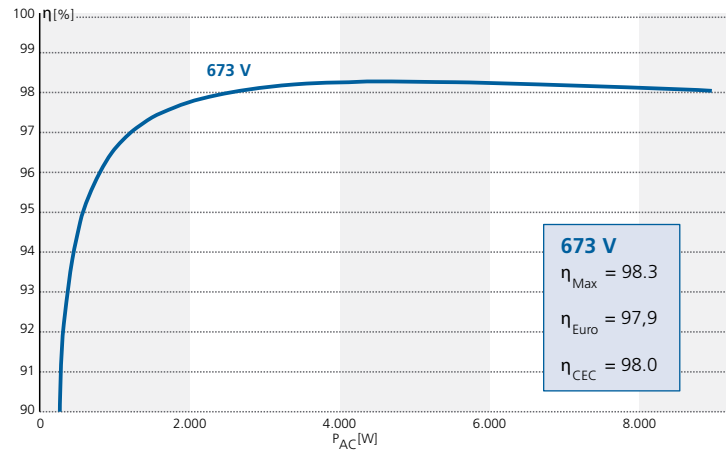
Wirkungsgradkennlinie Powador 9.0 TL3
